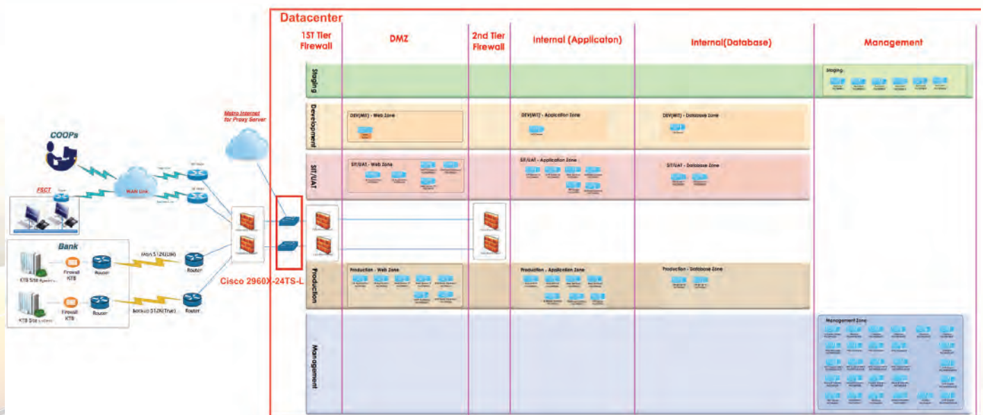
แผนผังแสดงการเชื่อมต่อของระบบ (Network Diagram)
